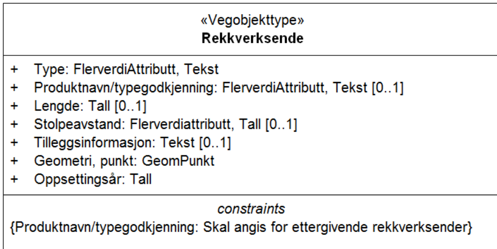
Figur 1: UML-skjema for Rekkverksende
