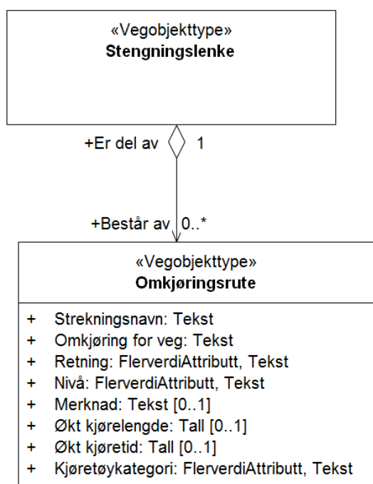
Figur 3: UML-skjema med assosiasjoner
