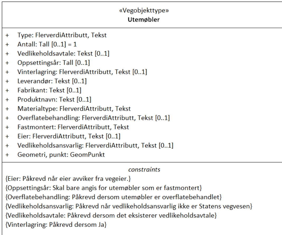
Figur 1: UML-skjema Utemøbler
