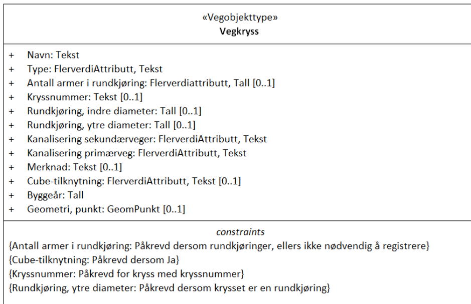
Figur 1:UML-skjema Vegkryss
