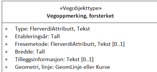
Figur 3: UML-skjema med assosiasjoner
