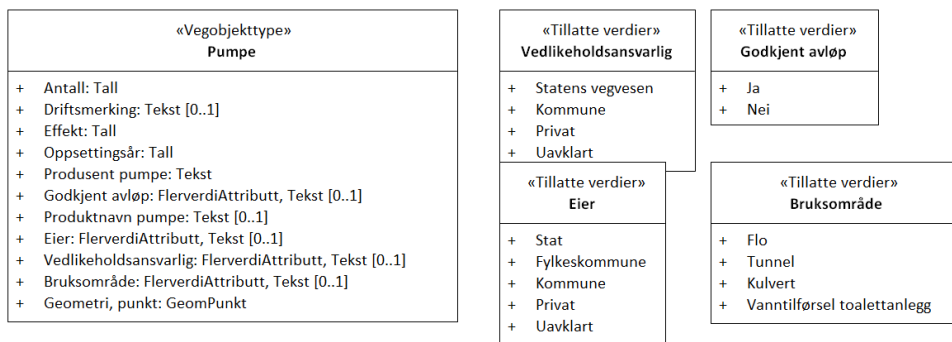
Figur 2: UML-skjema med tillatte verdier
