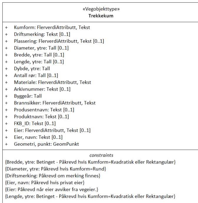
Figur 1: UML-skjema for Trekkefum
