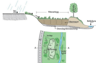
Figur 403.6. Utforming av åpent filterbasseng (plan/snitt)..
