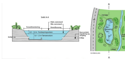
Figur 403.2 Uforming av vått overvannsbasseng
