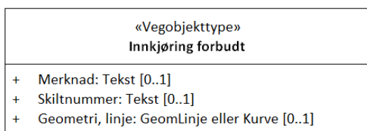
Figur 1: UML-skjema
