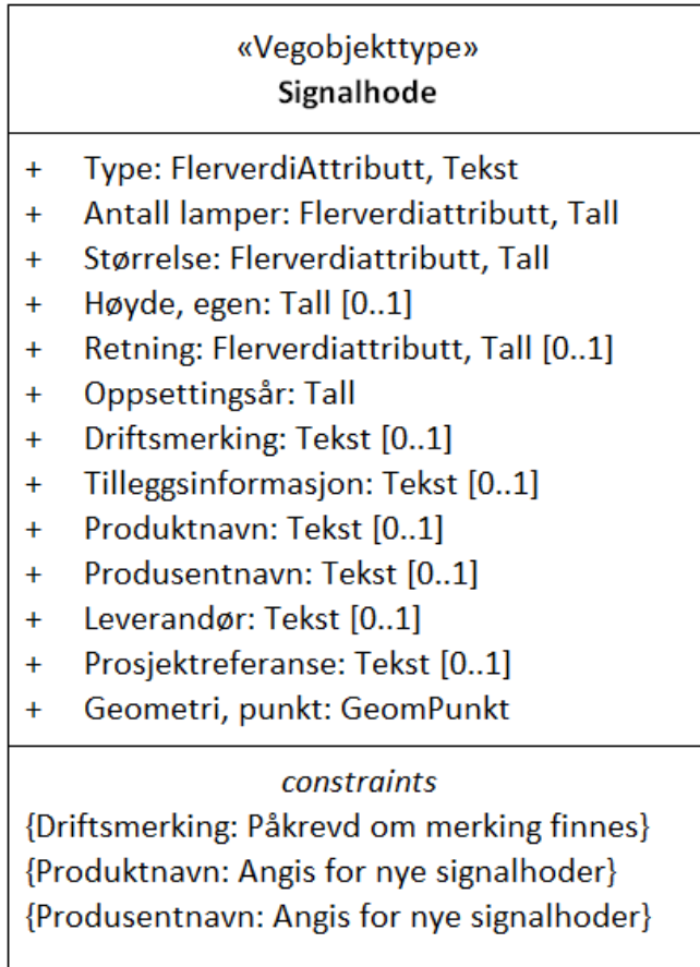
Figur 1: UML-skjema Signalhode
