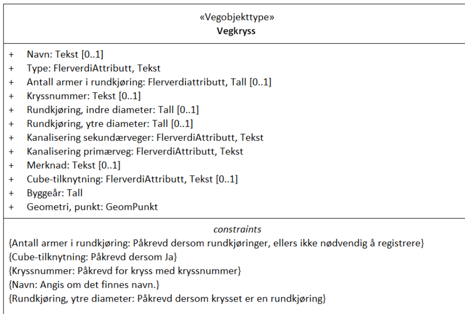
Figur 1:UML-skjema Vegkryss
